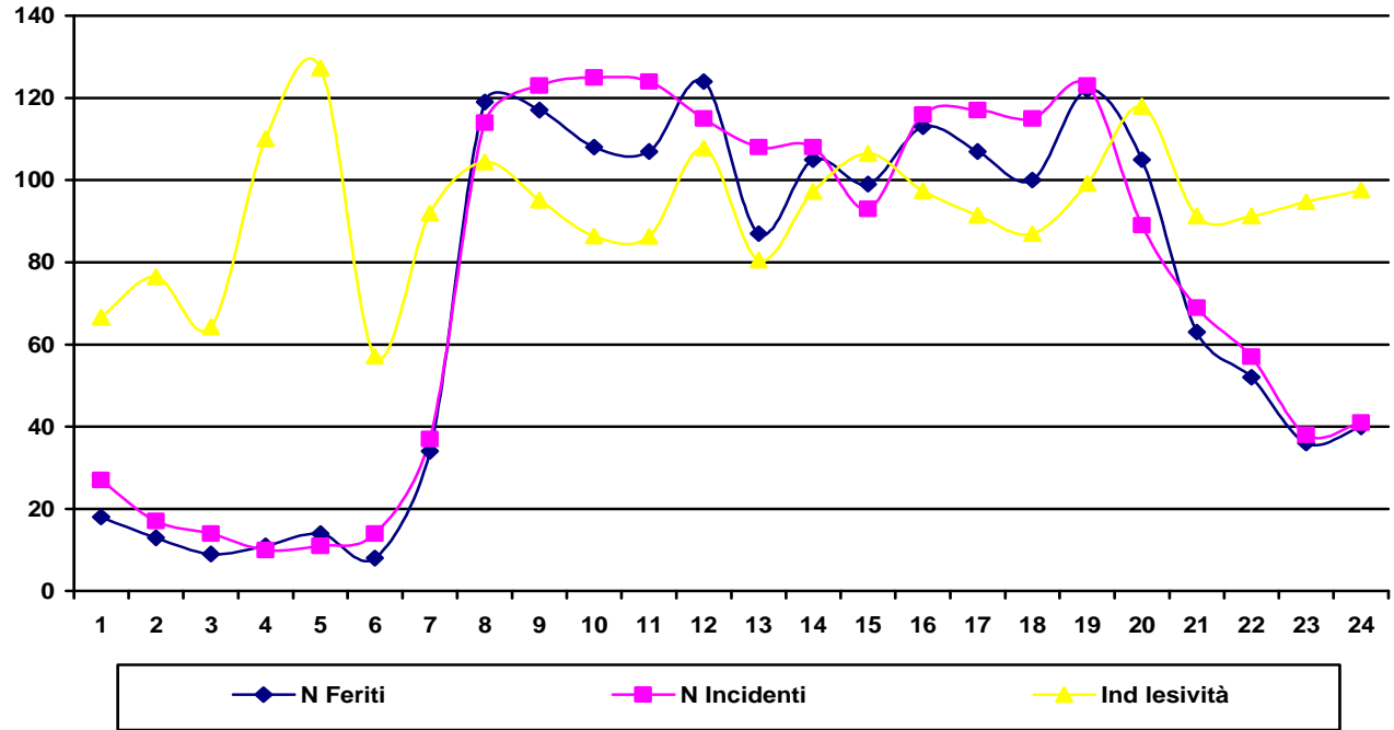
Numero di incidenti, feriti e indice di lesività per ora
